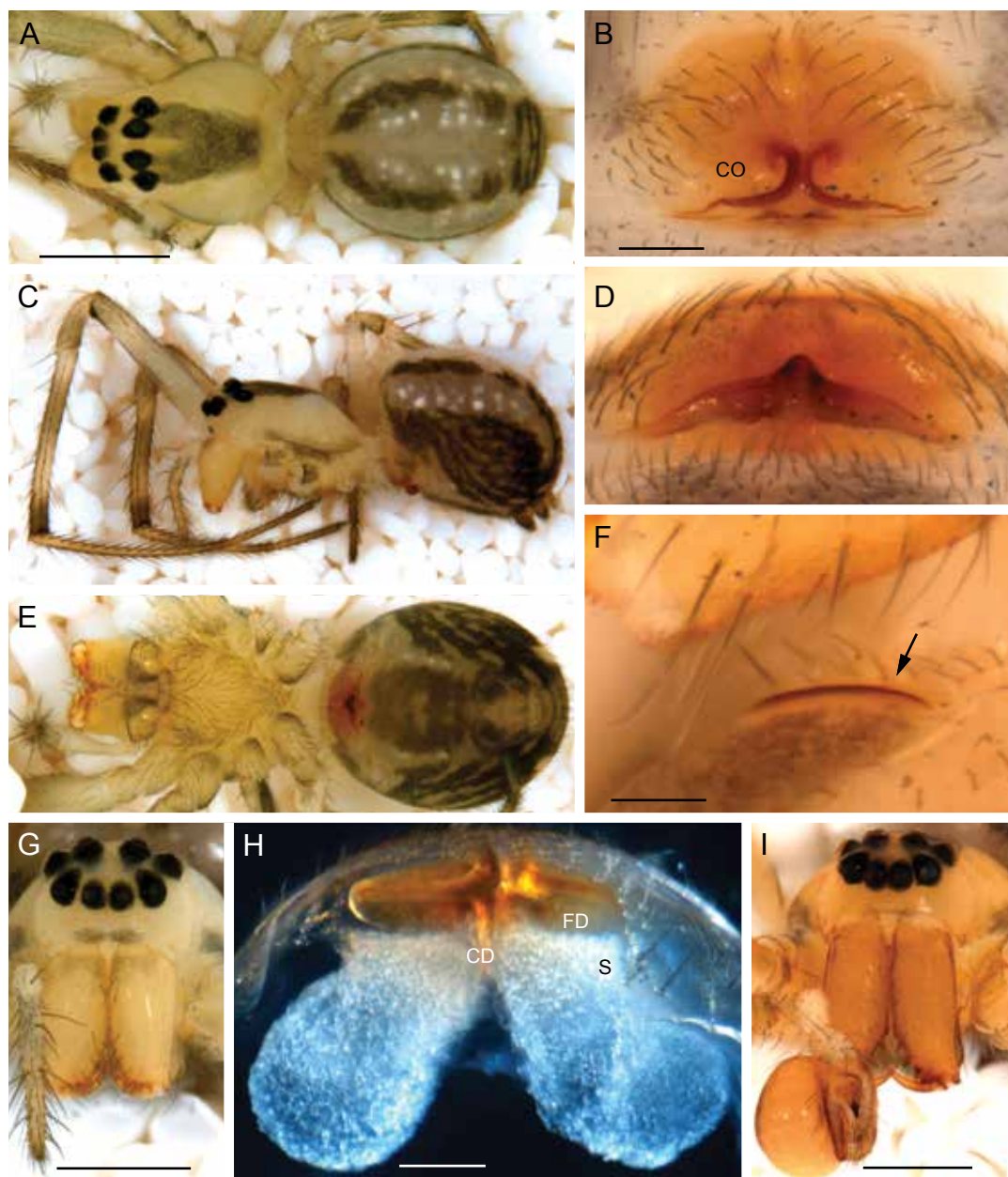
FIGURE 26. Nanometa purpurapunctata (TEAU025). A. Female, dorsal habitus. B. Epigynum ventral. C. Female, lateral habitus. D. Epigynum, caudal. E. Ventral habitus. F. Male, stridulatory organ. G. Female, frontal habitus. H. Epigynum, dorsal digested. I. Male, frontal habitus. Scale bars: A, C, E, 1.0 mm; B, D, F, H, 0.1 mm; G, I, 0.5 mm.
